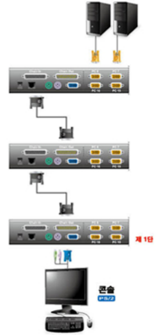
ACS1216A 16포트 KVM 스위치
