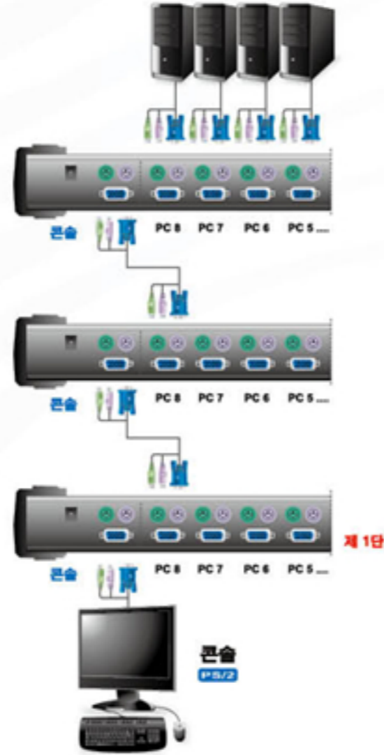
CS9138 8포트 KVM 스위치
